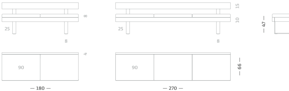
Sitzkissen 90 cm / Seat cushion 90 cm
