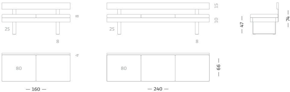
Sitzkissen 80 cm / Seat cushion 80 cm
