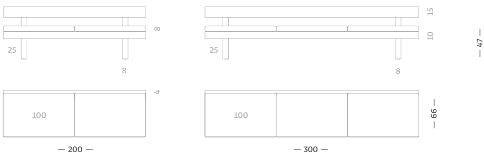
Sitzkissen 100 cm / Seat cushion 100 cm
