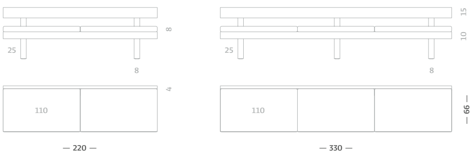
Sitzkissen 110 cm / Seat cushion 110 cm
